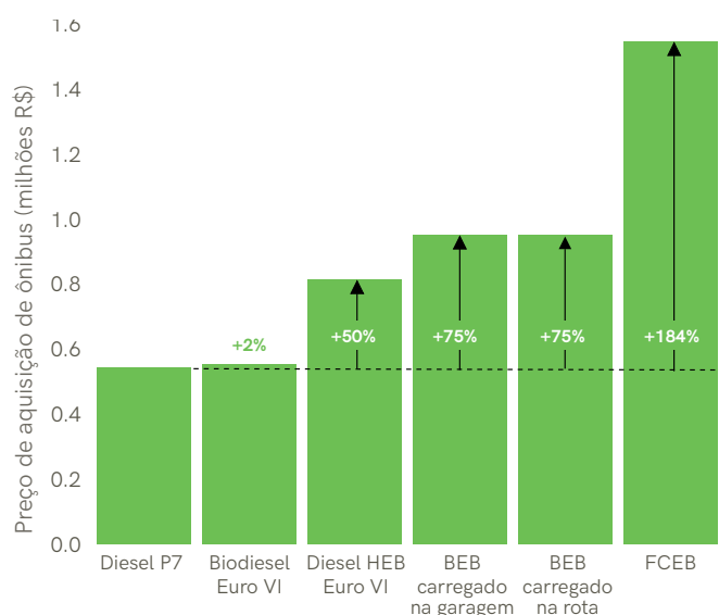
Figura 5-1 | Preço de compra de ônibus de transporte elétrico em comparação com ônibus convencionais a diesel 41
