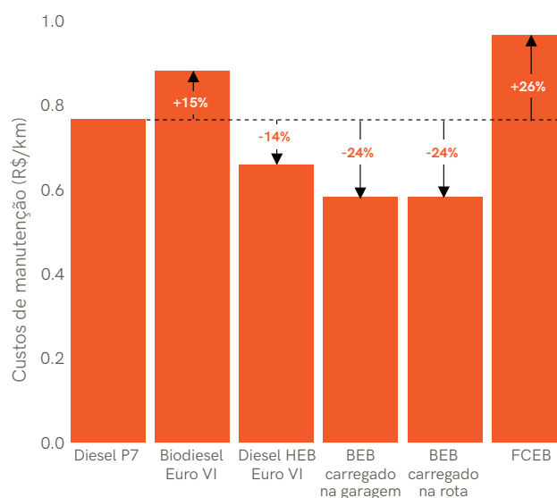
Figura 5-4 | Custos de manutenção de veículos regulares para ônibus de transporte elétricos em comparação com ônibus convencionais a diesel 44
