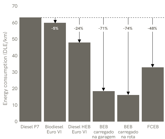
Figura 5-2 | Consumo de energia de ônibus de transporte elétricos em comparação com ônibus convencionais a diesel 42
