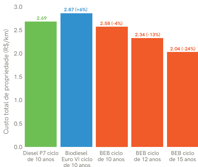
Figura 5-7 | Sensibilidade do TCO para um BEB Padron LE durante o período de propriedade 47
