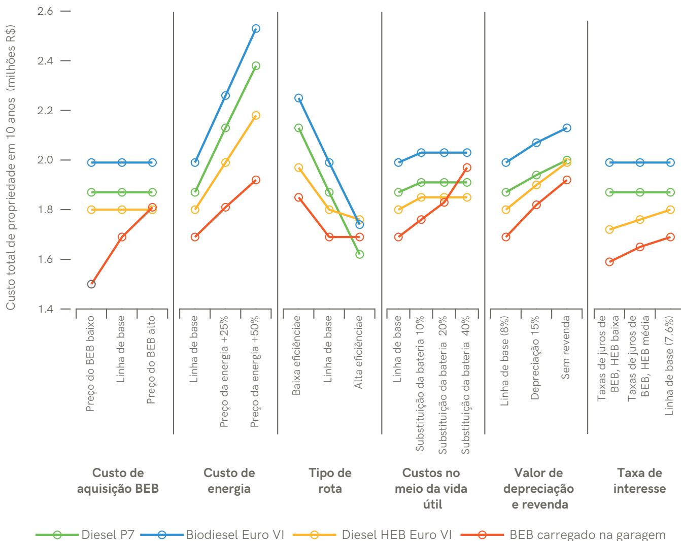
Figura 5-6 | Análise de sensibilidade para o TCO de um ônibus tipo Padron LE
