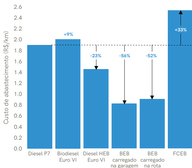
Figura 5-3. | Custos operacionais para ônibus com tecnologia alternativa em comparação com ônibus convencionais a diesel 43
